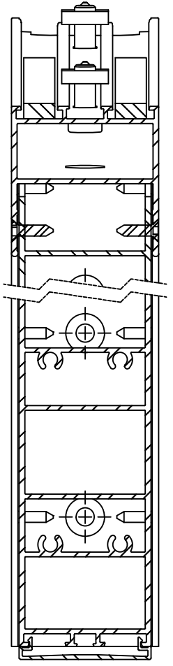
B-B (1 : 1)
