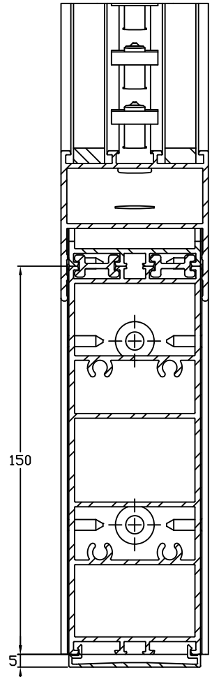
A-A (1 : 1)
