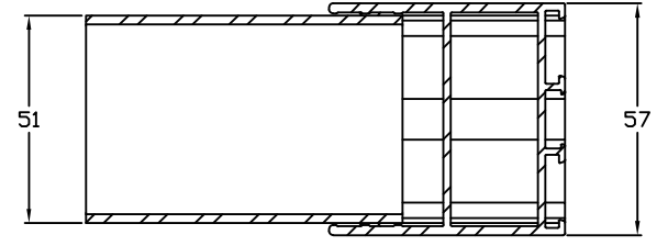
D-D (1:1)
