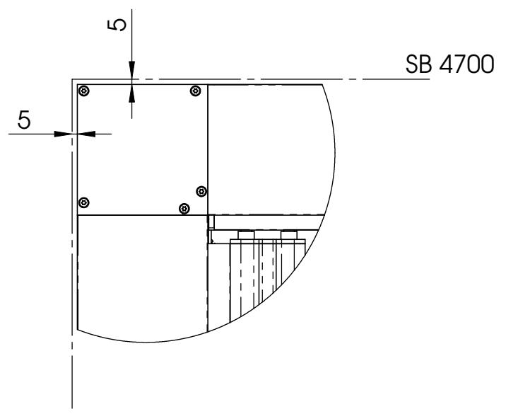
DETAIL H MAßSTAB 1 : 5
