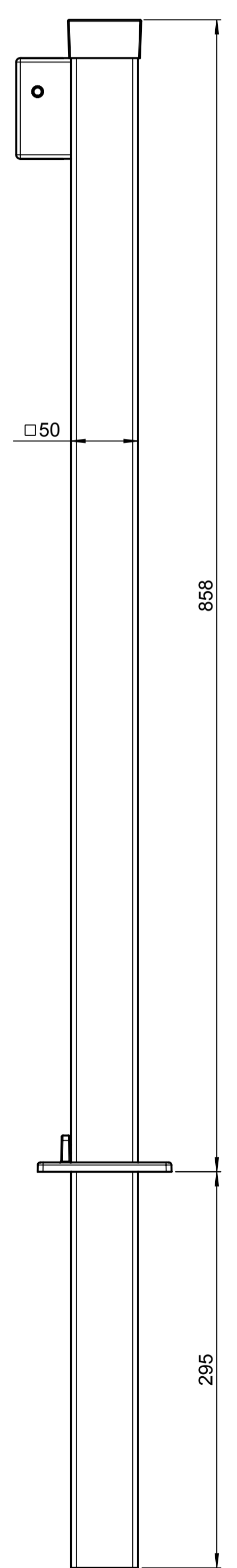
Einsteckpfosten SR414/2
