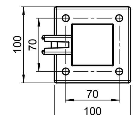
Aufsraubpfosten SR415/1
