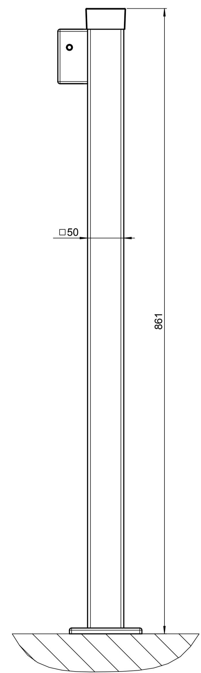
Aufsraubpfosten SR415/1
