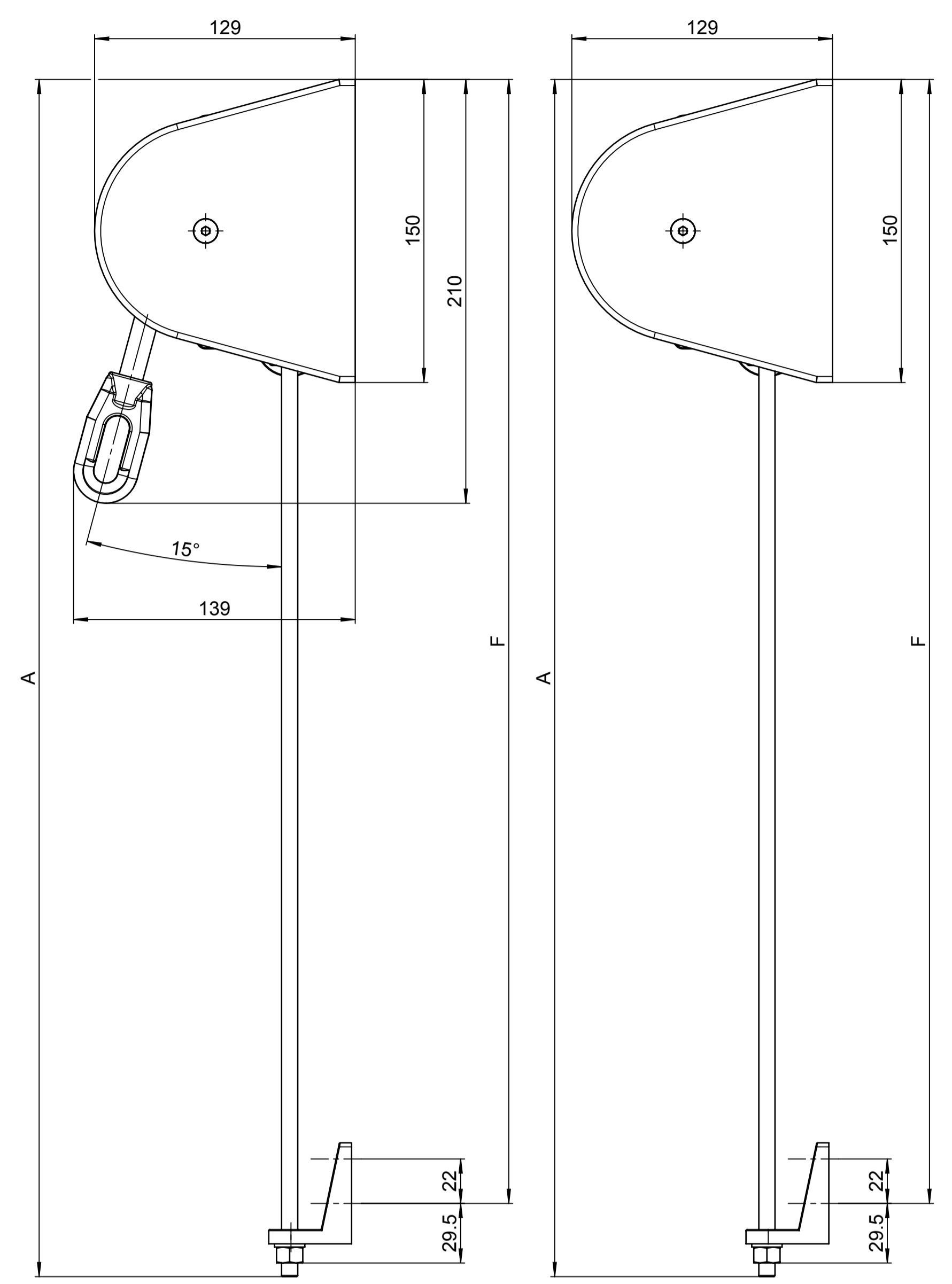
mit Getriebe
