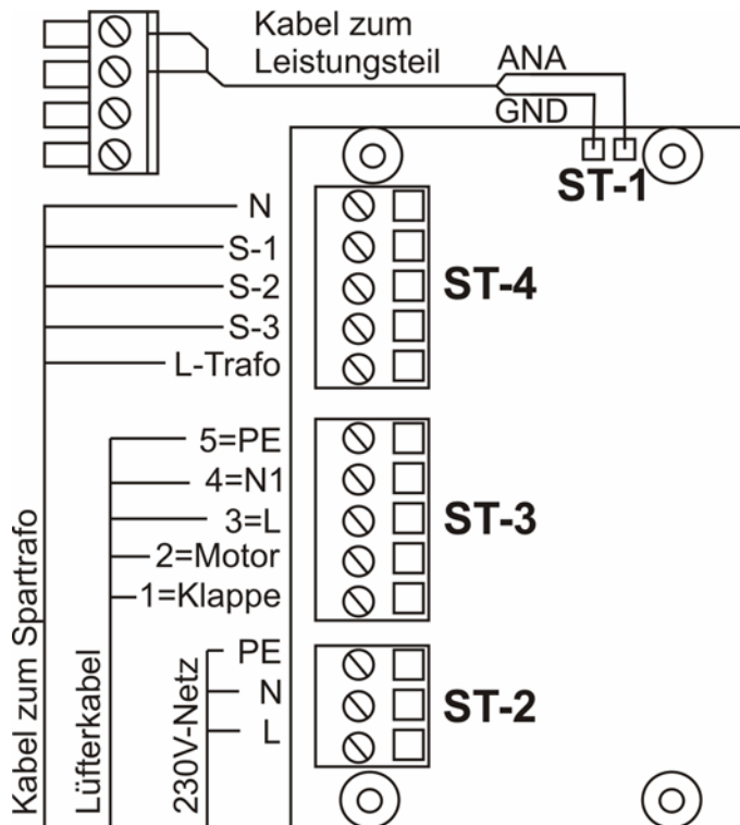
Bild 6: Steckerbelegung der 4-Stufen-Regelplatine
