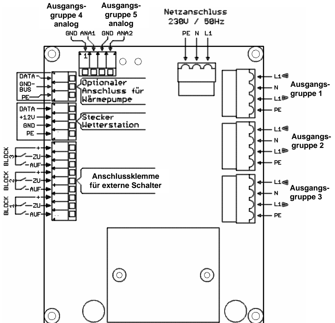
Bild 3: Steckerbelegung (3 bis 5 Ausgangsgruppen)
