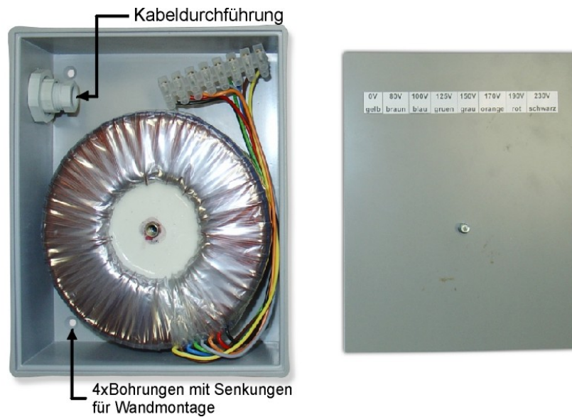
Bild 7: Spartrafo anschließen
