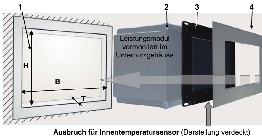
Bild 1: Montagereihenfolge für Einbau unter Putz mit Unterputzgehäuse
