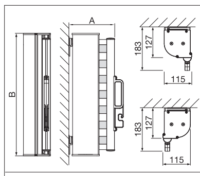
SR6000 Wandmontage / Plafondmontage
