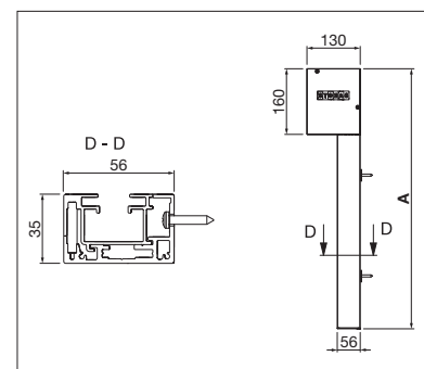
VS6200 Montage mural par vissage direct
